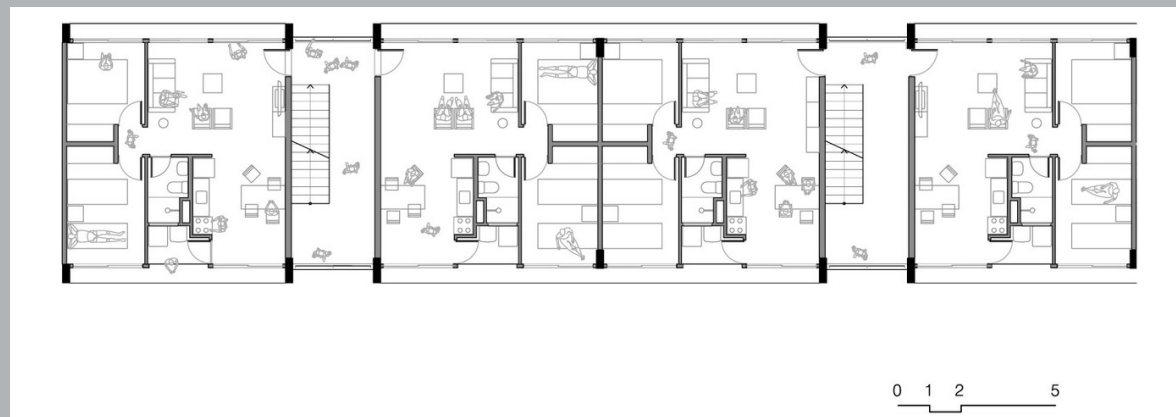
Planta Tipo - Edifício Edite 2 e 5
