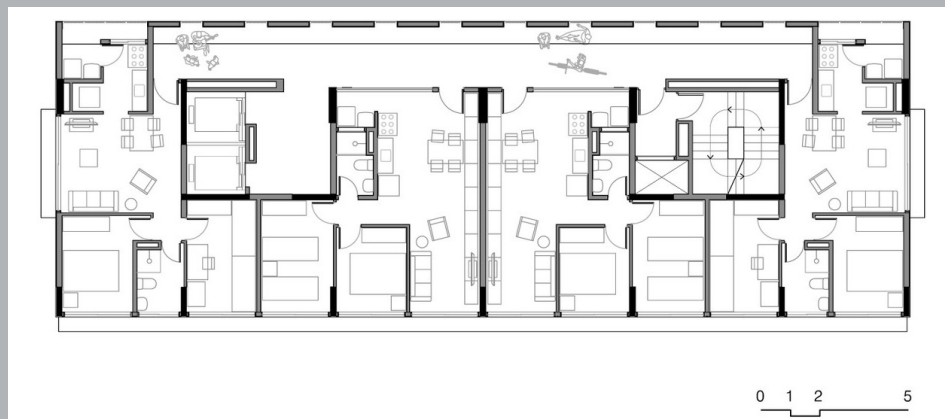
Planta Tipo - Edifício Edite 1, 3 e 4
