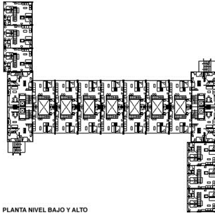
PLANTA NIVEL BAJO Y ALTO
